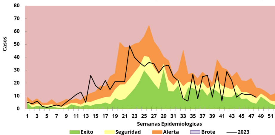
Corredor endémico semanal de Bronquiolitis menores de 2 años. Provincia de Tierra del Fuego - hasta SE 48 - Año 2023 Históricos 5 años: 2015 a 2019. (excluido años 2020-2021-2022)
